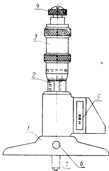
1 — основание; 2 — стембель; 3 — барабан; 4 — трещотка (фрикцион); 5 — табло циф- рового устройства; 6 — стопор; 7 — изме- рительный стержень
