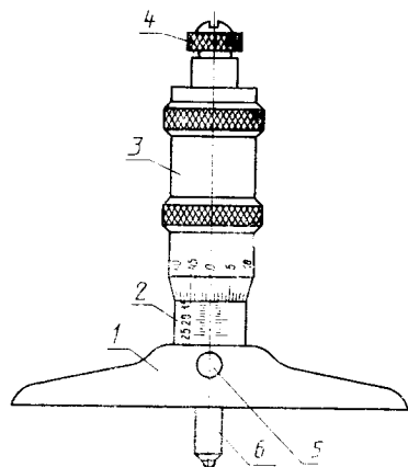
1 — основание; 2 — стембель; 3 — барабан; 4 — трещотка (фрикцион); 5 — стопор; 6 — измерительный стержень
